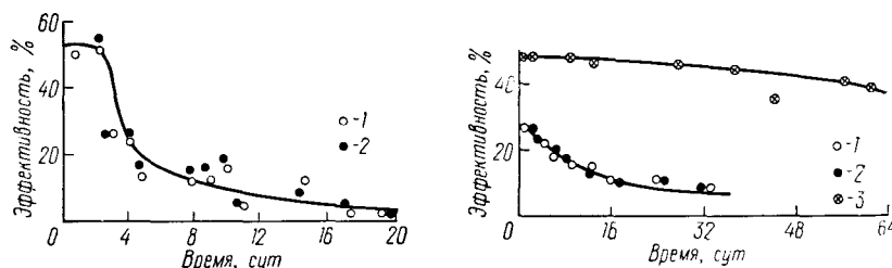
Рис. 1. Эффективность депрессора испарения в зависимости от времени: 1 — в кюветах с кристаллами депрессора испарения на дне; 2 — в кюветах с пленкой депрессора испарения.
